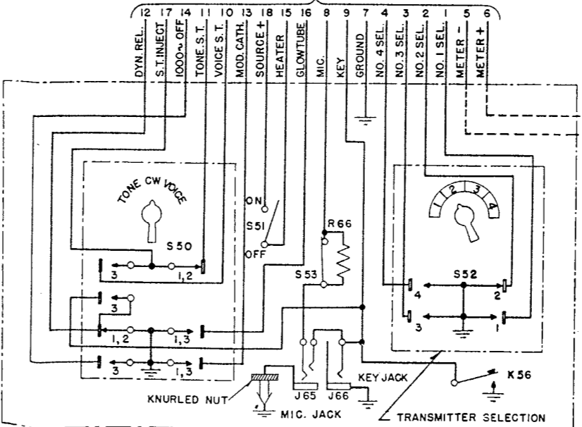
RADIO CONTROL BOX BC-451-A
